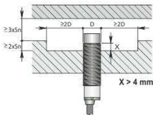
Montaggio spogente
